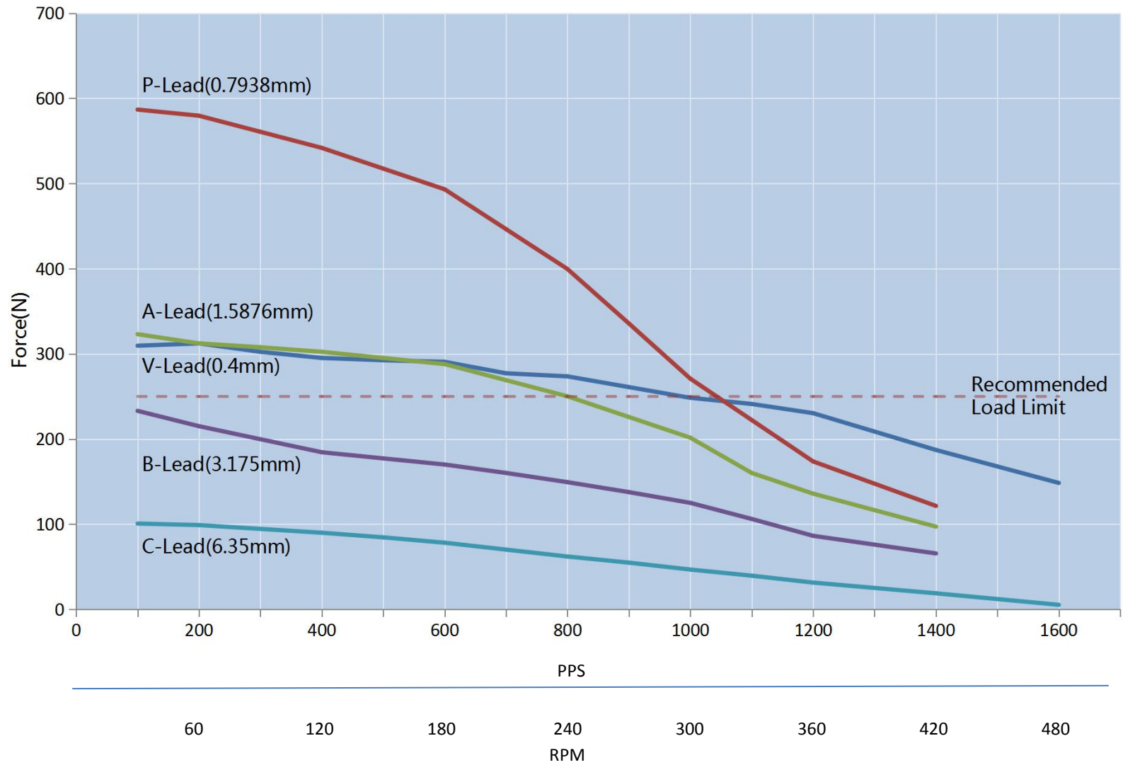
Nema 17 linear steppers(24V)
